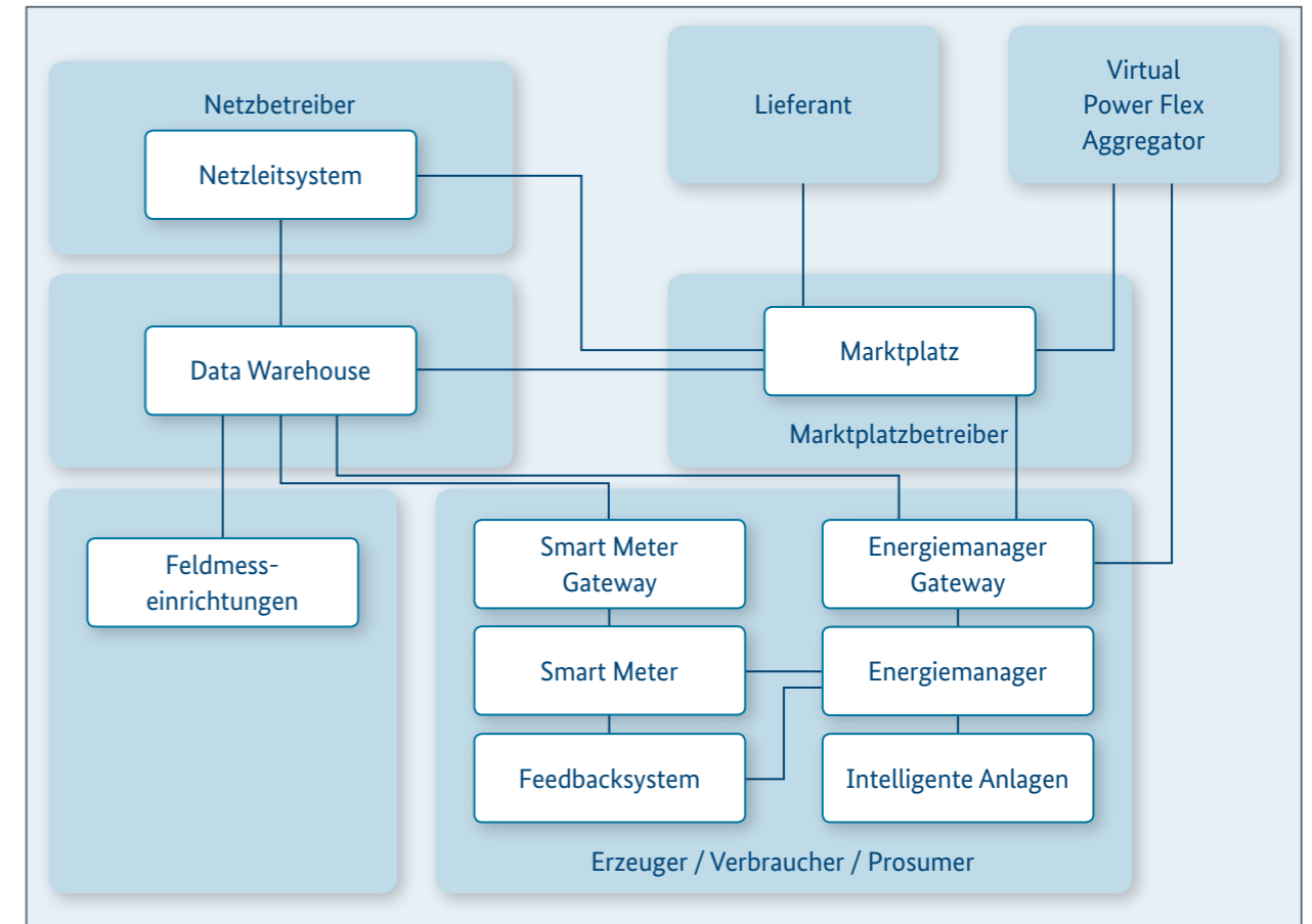
Komponenten im Internet der Energie (Variante 0)
