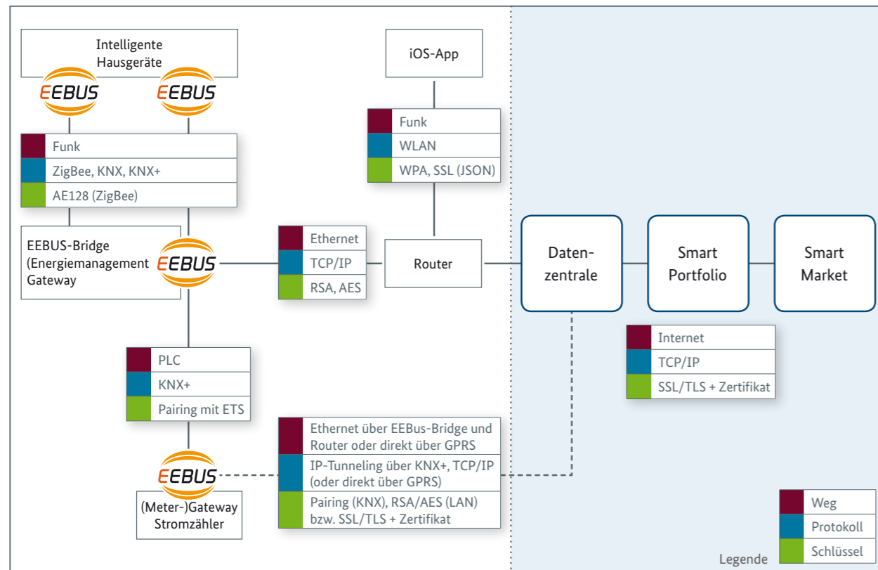
Systeme und Komponenten im Smart-Watts-Feldversuch
